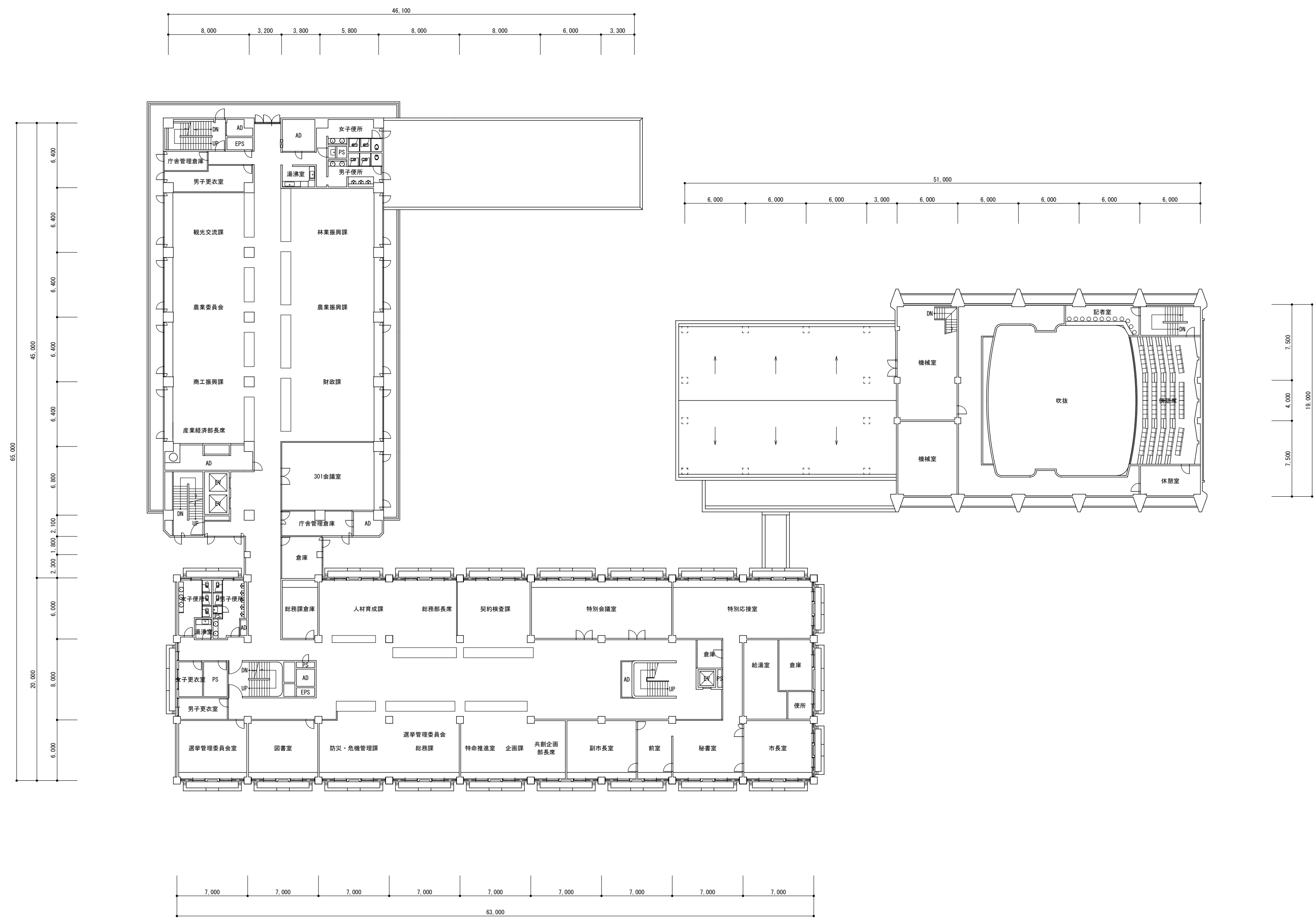
3 階平面図
