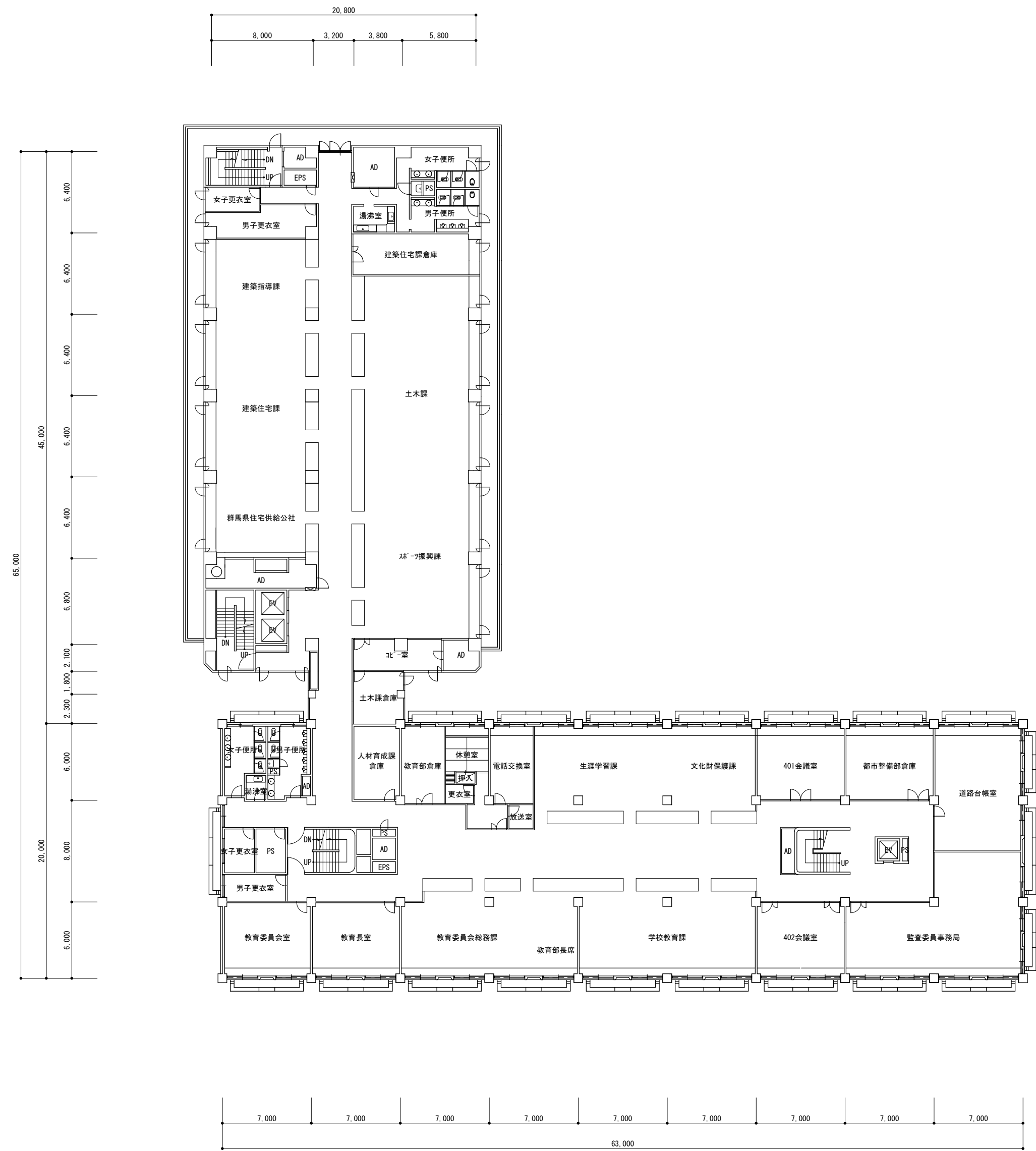
4 階平面図
