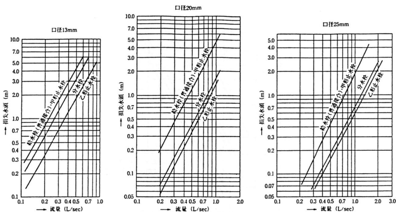
図－3．5－1 水栓類の損失水頭例（給水栓、止水栓、分水栓）
