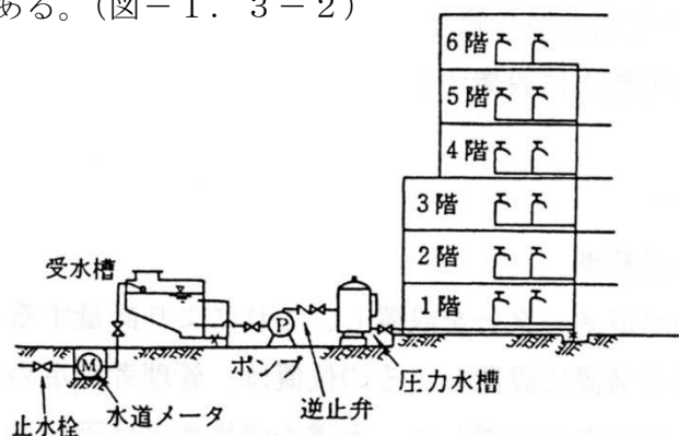
図－１．３－２ 圧力水槽式
