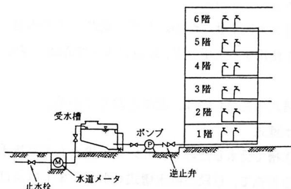
図－１．３－３ ポンプ直送式
