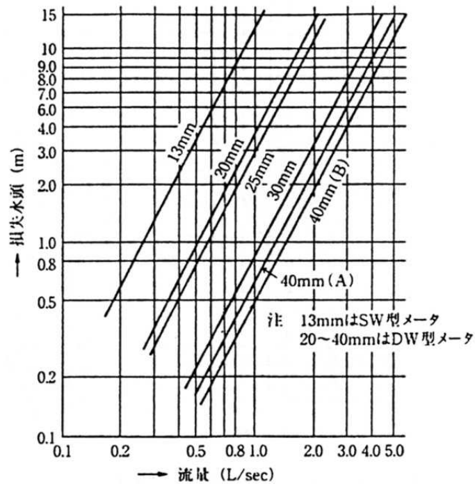
図-3.6 メータの損失水頭例
