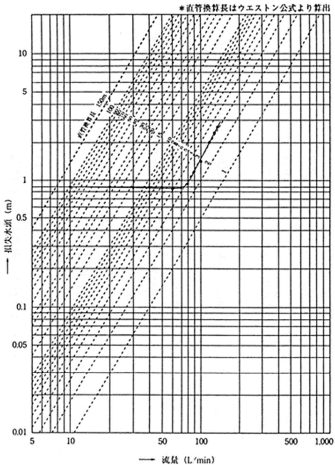
図一 3.5 - 2 水栓類の損失水頭例（呼び径 25 単式逆止弁）
