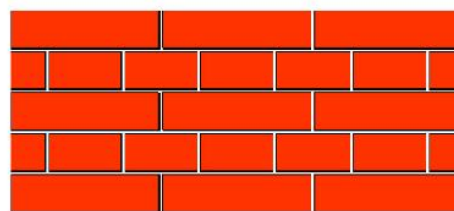
イギリス積み
