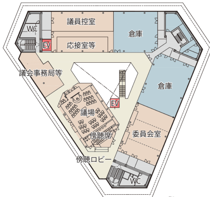
4階平面図
