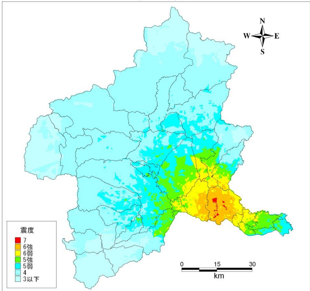
太田断層による地震 (M7.1)
