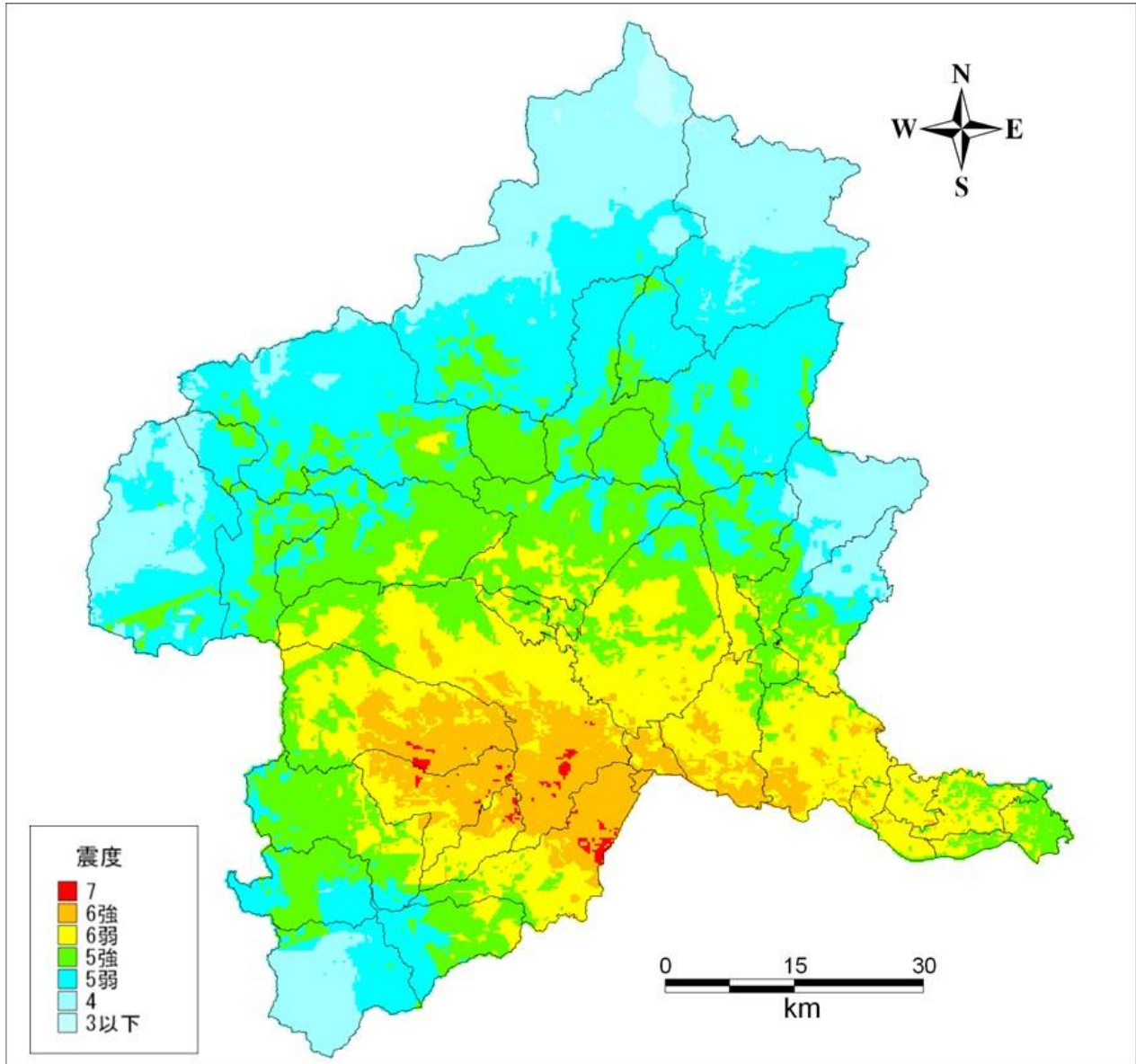
関東平野北西縁断層帯主部による地震 (M8.1)
